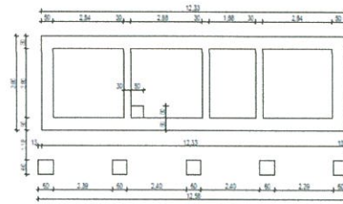
Alapozási alaprajz
