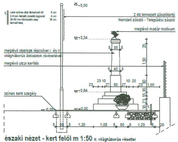
északi nézet - kert felől m 1:50 II. világháborús vésettel
