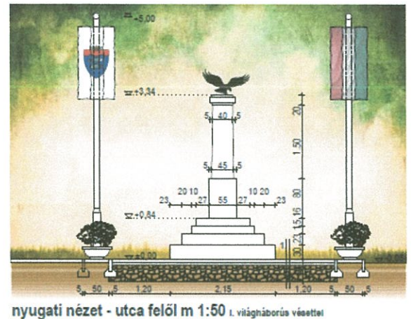
nyugati nézet - utca felől m 1:50 I. világháborús vésettel
