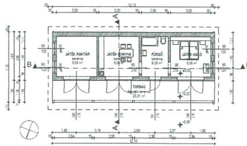
Földszinti alaprajz
